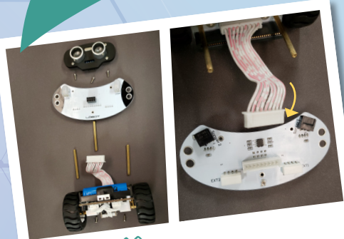
擰上螺絲
